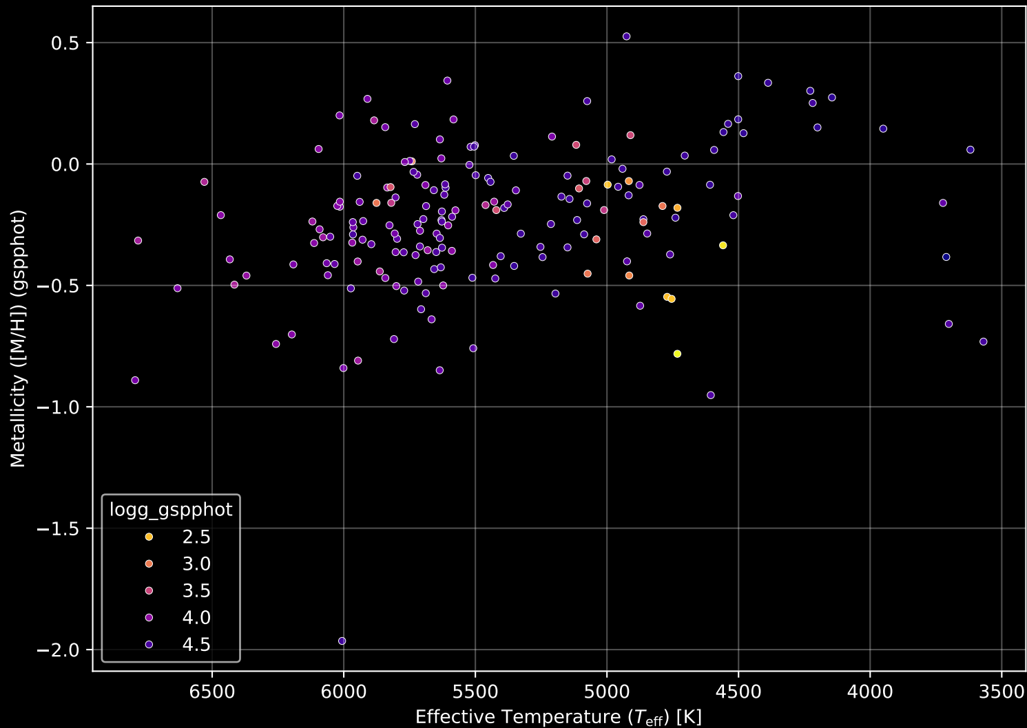
APOGEE DR17 Field: [133+76_MGA] Stellar Population Parameters (n= 183)
